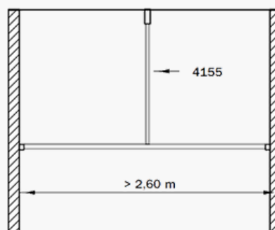
Montage avec naissance et montant de plafond
