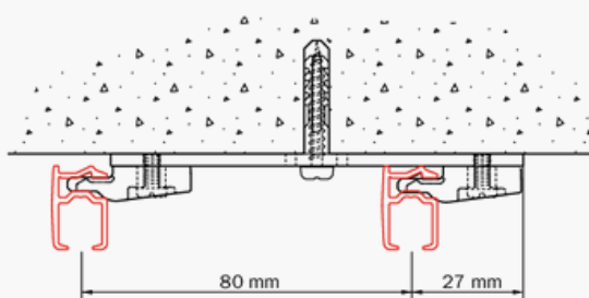
Montage double plafond avec supports 5350
