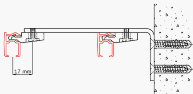
Montage mural avec équerre 2015
