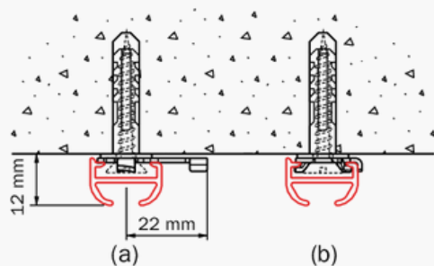
Montage plafond avant(a) et après(b) serrage support 2650
