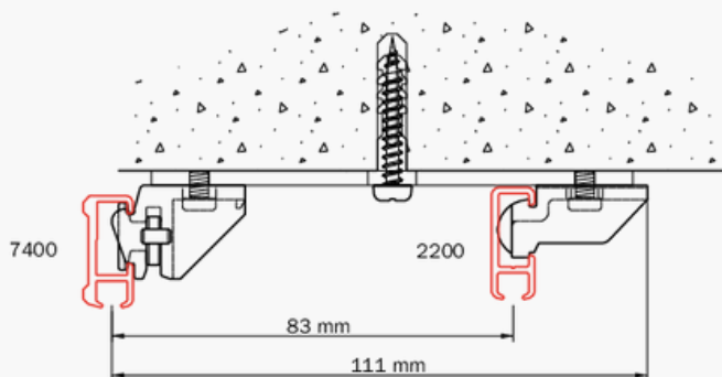
Montage double au plafond avec 2216 et support 7450 et 2250
