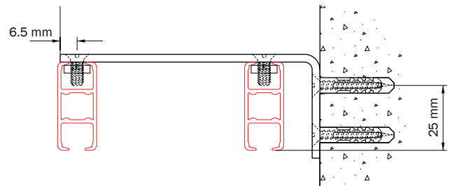
Montage avec équerre 4115
