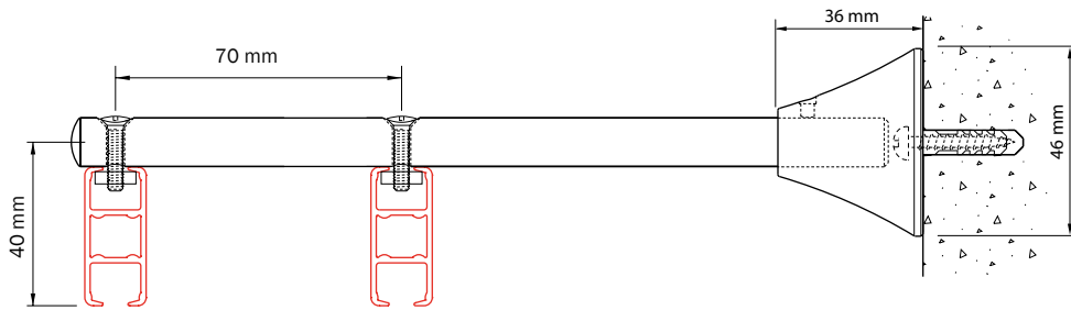
Montage avec équerre réglable
