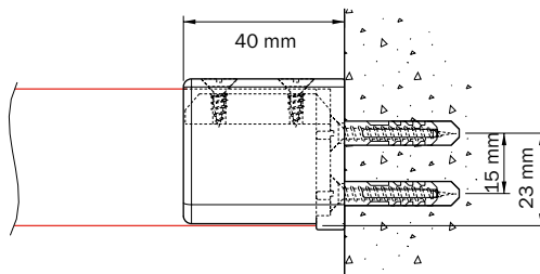
Montage au mur avec support 4149
