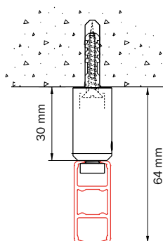
Montage au plafond avec bobine de plafond 4254
