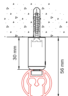
Montage au plafond 5100 avec montant de plafond 4254
