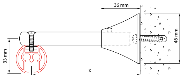
montage au mur avec équerre raccourcissable 4217-101, le support peut être raccourci jusqu'à x = 50\text{mm}
