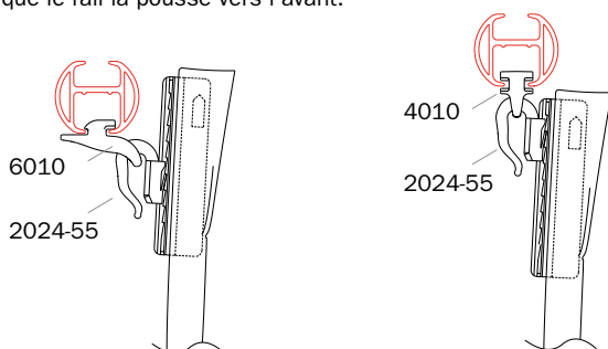
Tête de rideau avec glisseur décalé 6010 largeur 15 mm
